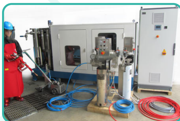
Esempio di impianto completo di componenti speciali forniti come optional
